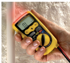
Kontaktlose Spannungsprüfung
