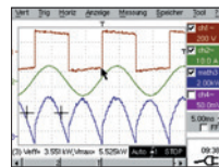
Wenn zwei Kanäle multipliziert werden, können das skalierte Ergebnis mit seiner physikalischen Einheit (z.B. W) und die Ausgangskurve optisch angezeigt werden, in diesem Fall Strom und Spannung.
