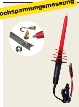
Hochspannungstastkopf SHT 40 kV für Multimeter
