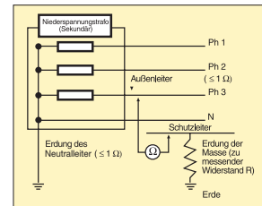
Prinzip der Schleifenwiderstandsmessung / Neutralleiter liegt auf Erde
